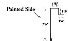
OVERHEAD DOOR JAMB
