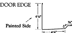
DOOR EDGE
