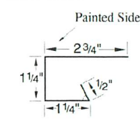
JAMB TRIM
