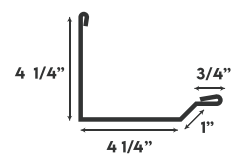
DOOR EDGE
