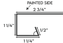
JAMB TRIM
