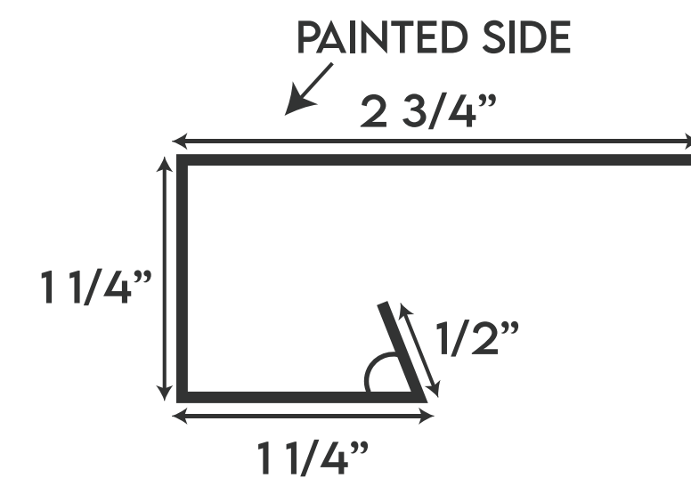
JAMB TRIM
