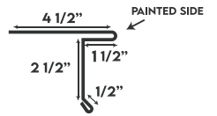
DRIP EDGE
