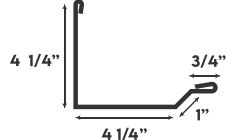
DOOR EDGE
