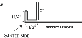
OVERHEAD DOOR JAMB
