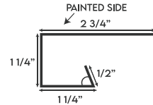
JAMB TRIM
